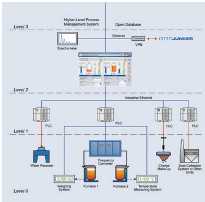
JOKS diagram
